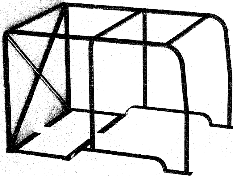
Figura 1 – Geometria de la estructura antivuelco
